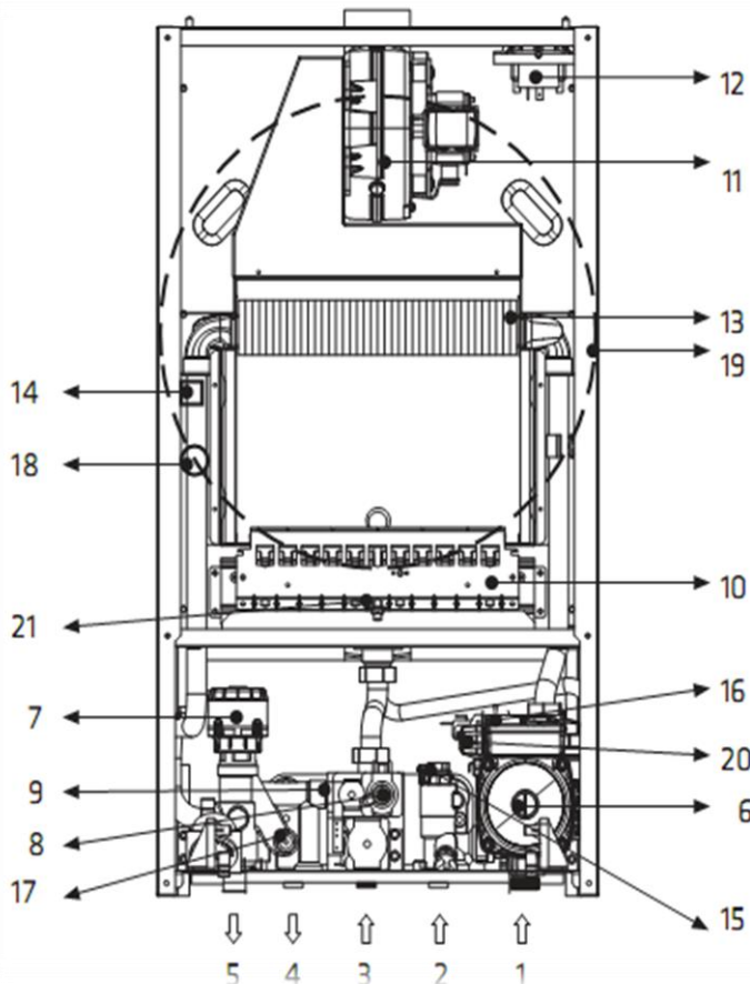
Рис 3. Монтажные соединения.
