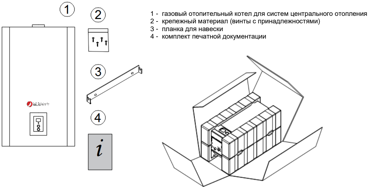
Рис 1. Комплект поставки.
