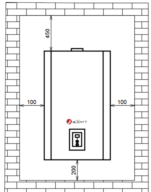
Рис 7. Установка в нише.
