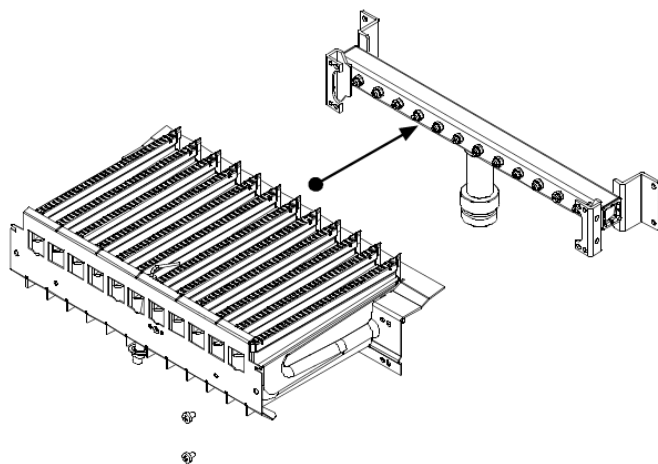
Рис 18. Смена типа газа.
