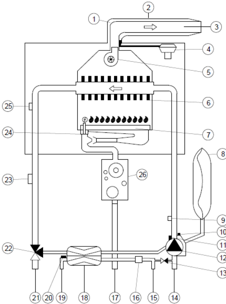
Рис 5. Функциональная схема.
