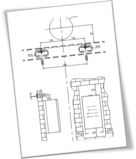
Рис 9. Монтажный шаблон.
